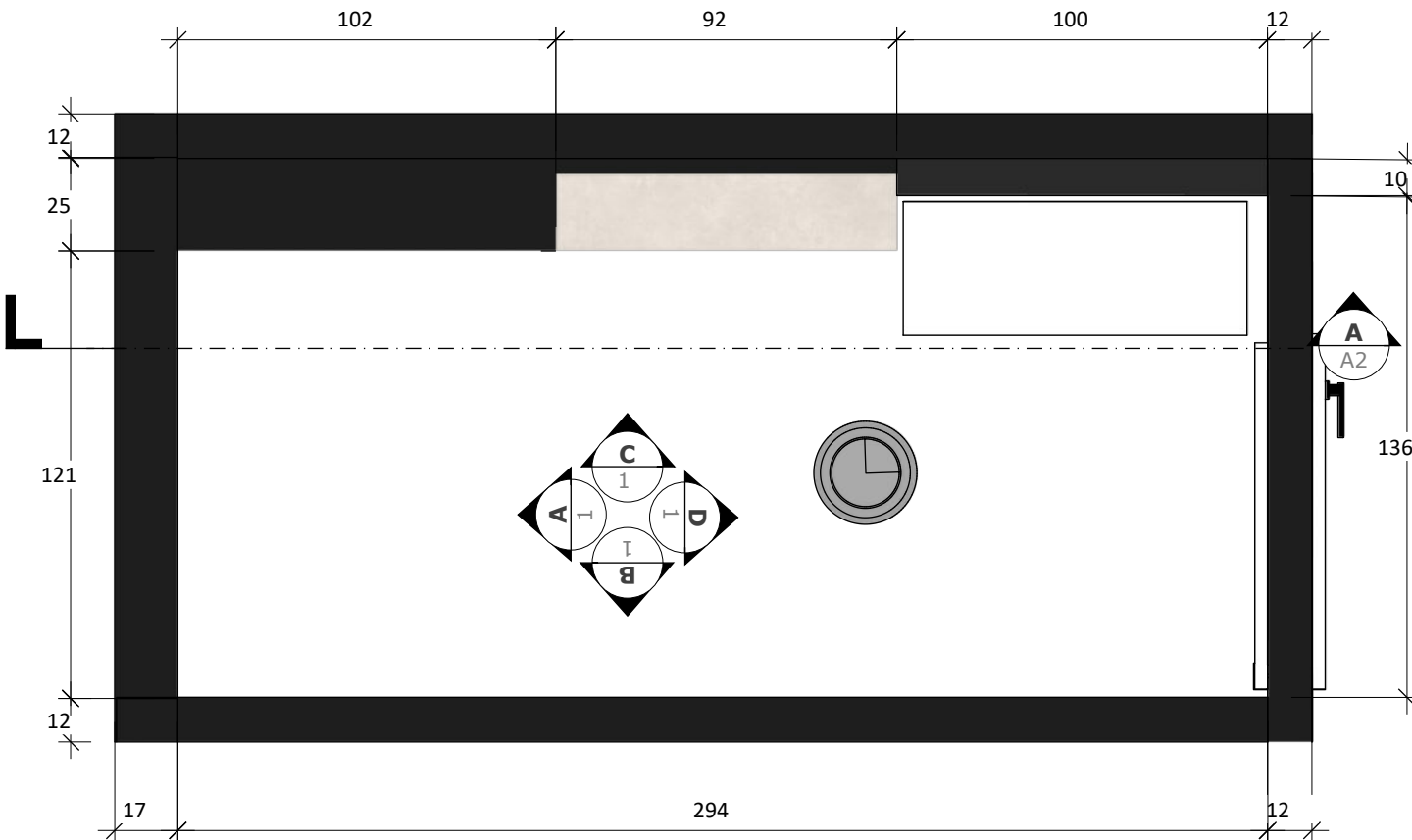
A :: Plan namještaja - Mala kupaonica 01 M 1:20
