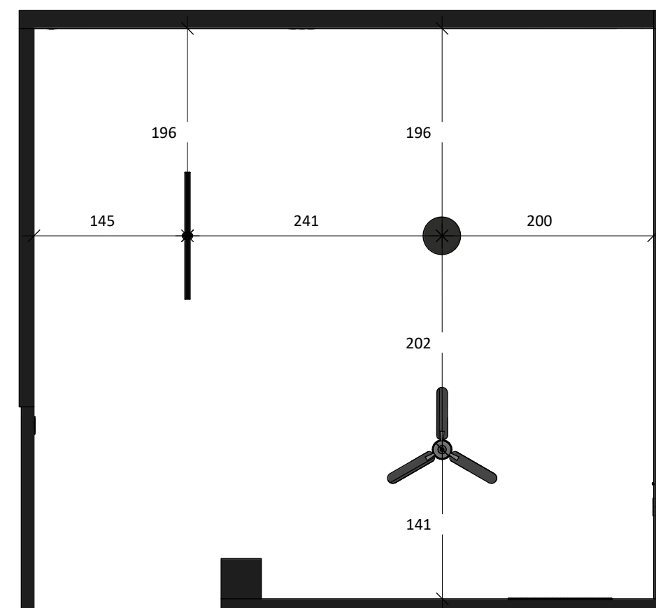
A :: Plan rasvjete - Dnevni boravak i blagovaonica 002 M 1:50
