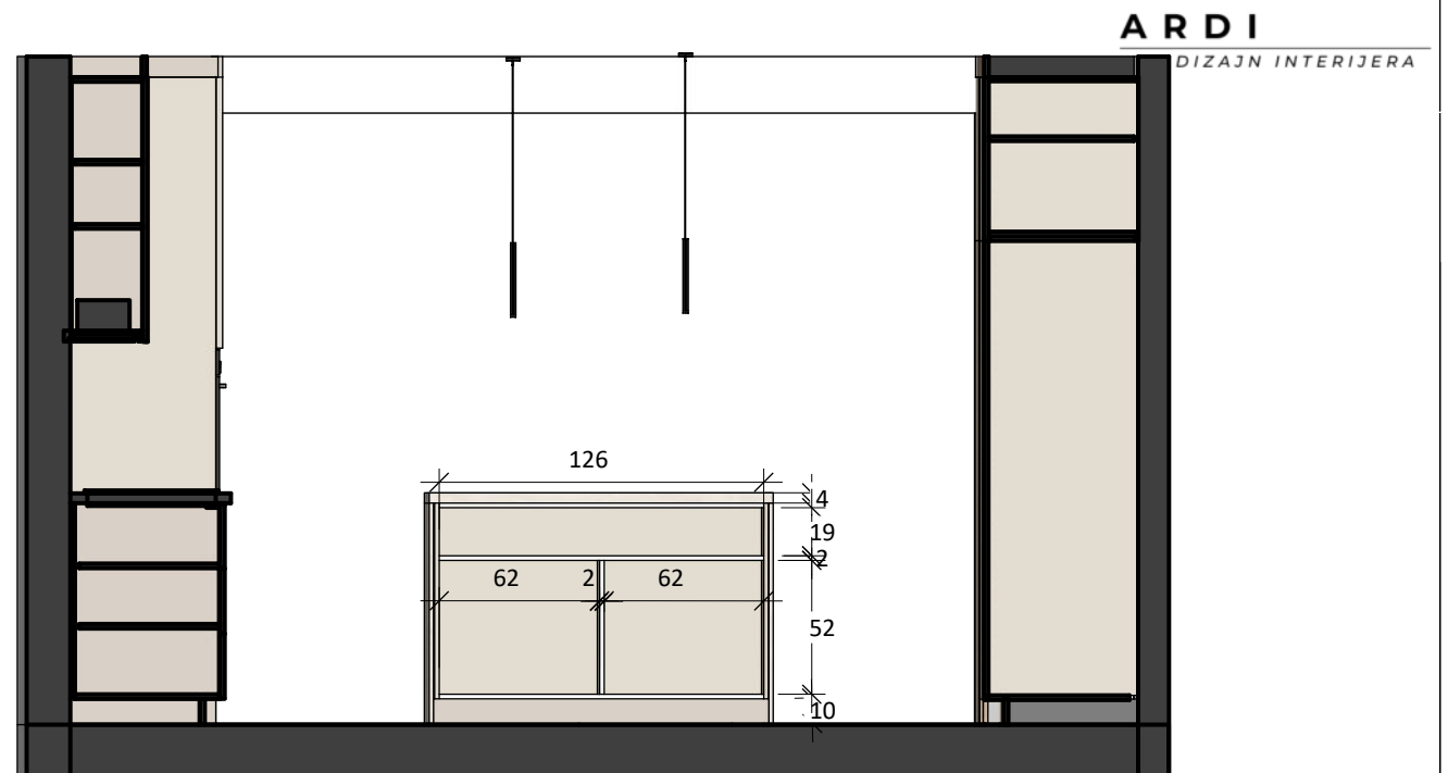
A :: Kuhinja - pogled prema dnevnom boravku 02 M 1:32
