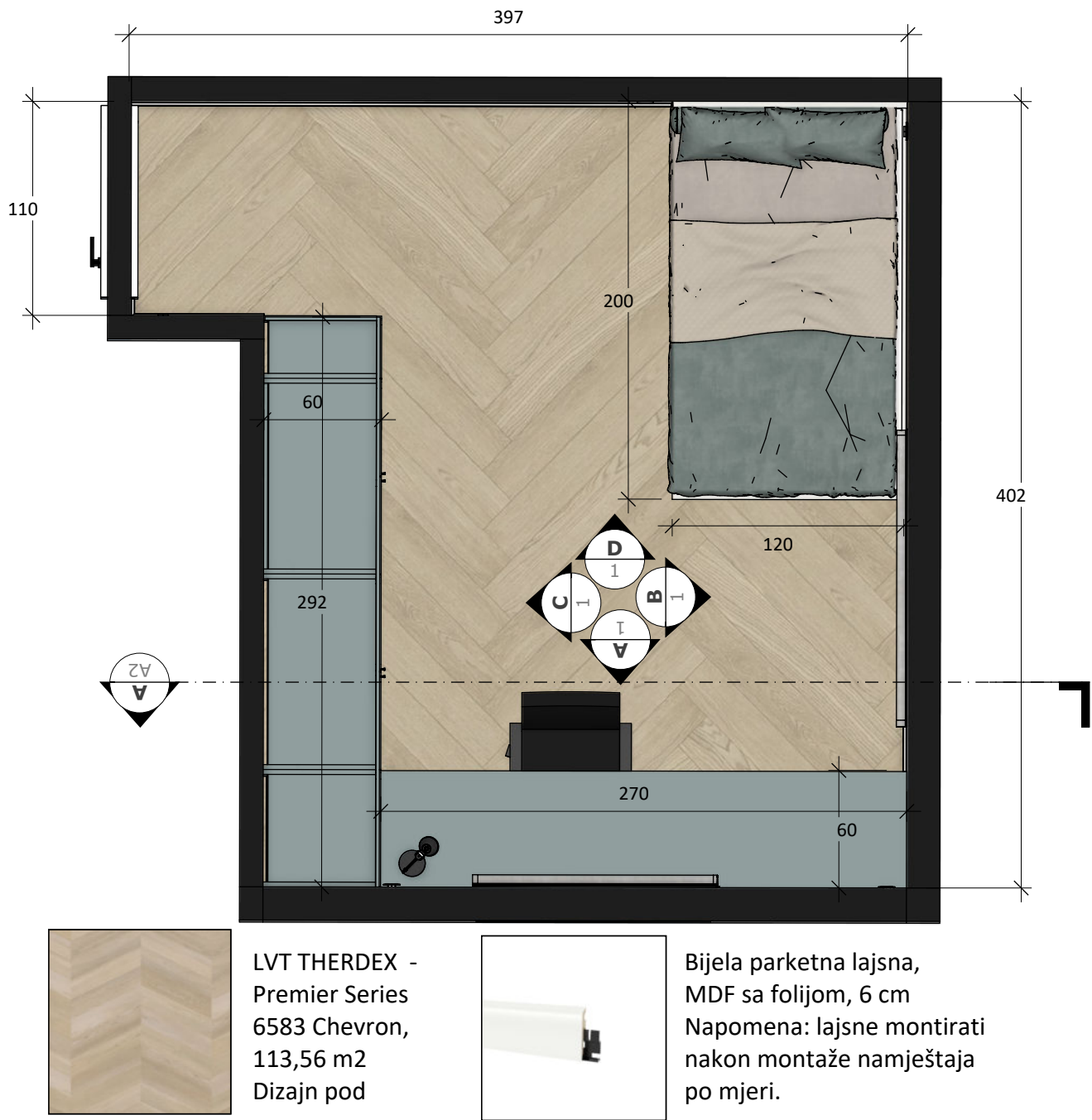
A :: Plan namještaja - Dječja soba I 01 M 1:32
