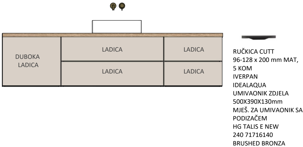
03 :: Velika kupaonica - ormarić s umivaonikom M 1:20
