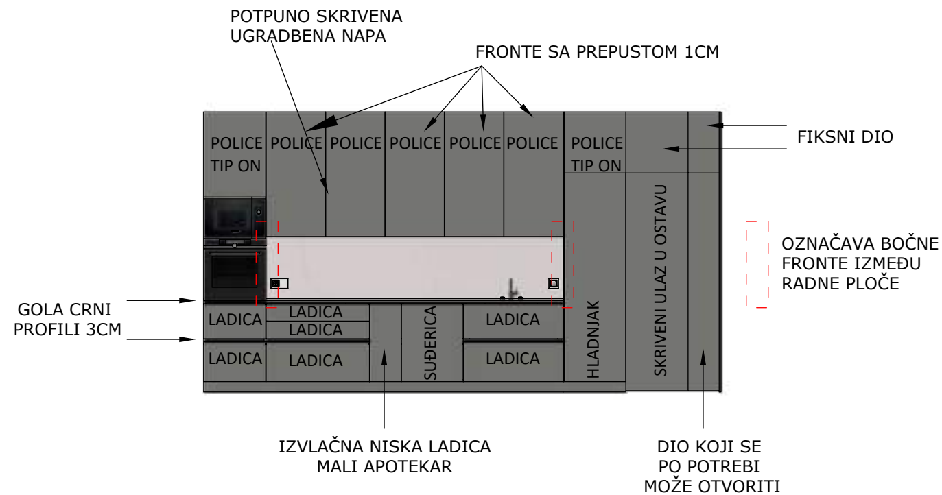
A :: Kuhinja - pogled na desno 01 M 1:50
