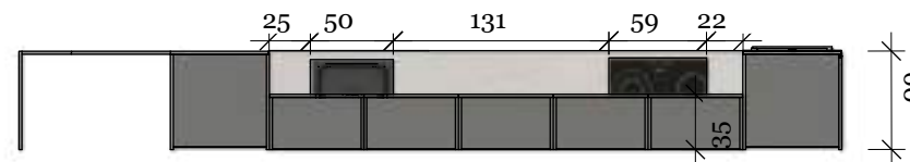
A :: Kuhinja - pogled sa strane 03 M 1:50
