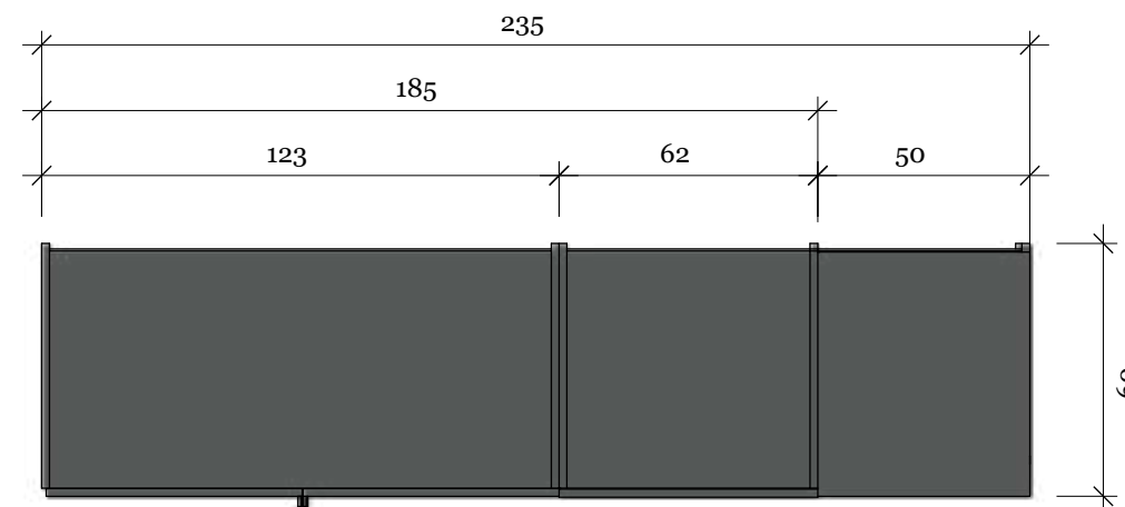
A :: Ormar - pogled odozgo 02 M 1:20
