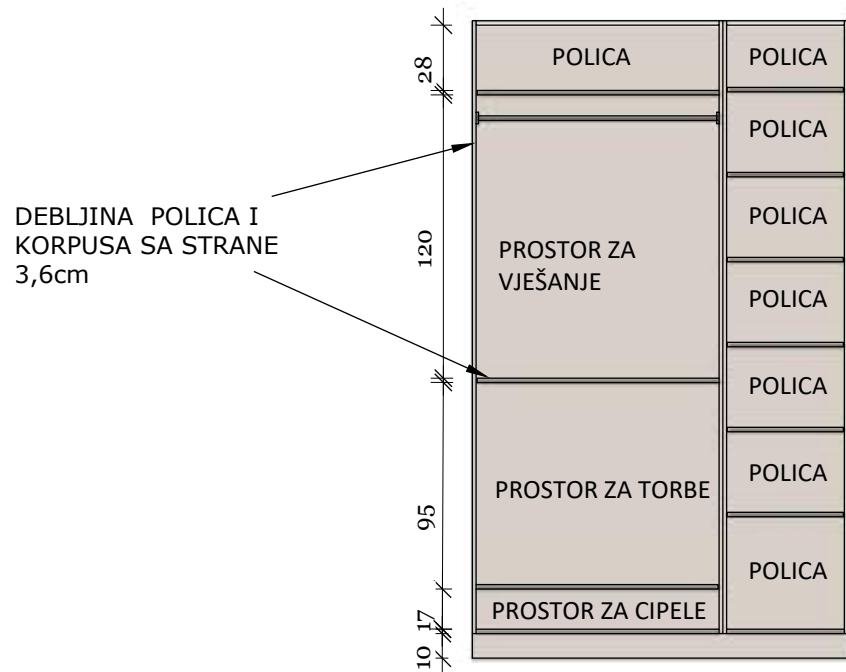
A :: Ormar u spavaćoj sobi skica 03 M 1:32
