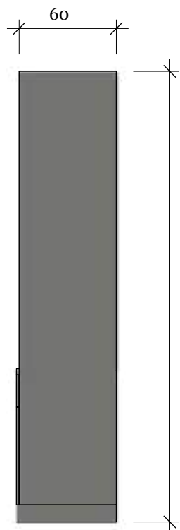
A :: Ormar - pogled sa strane 04 M 1:32
