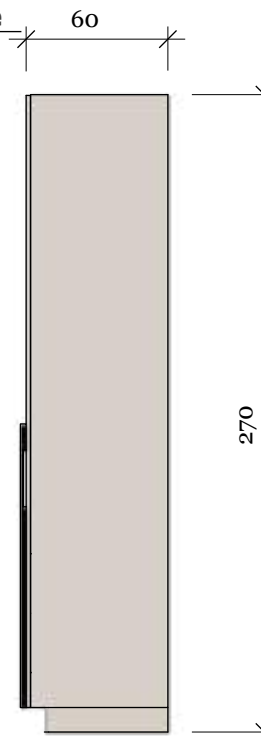
A :: Ormar - pogled sa strane 04 M 1:32
